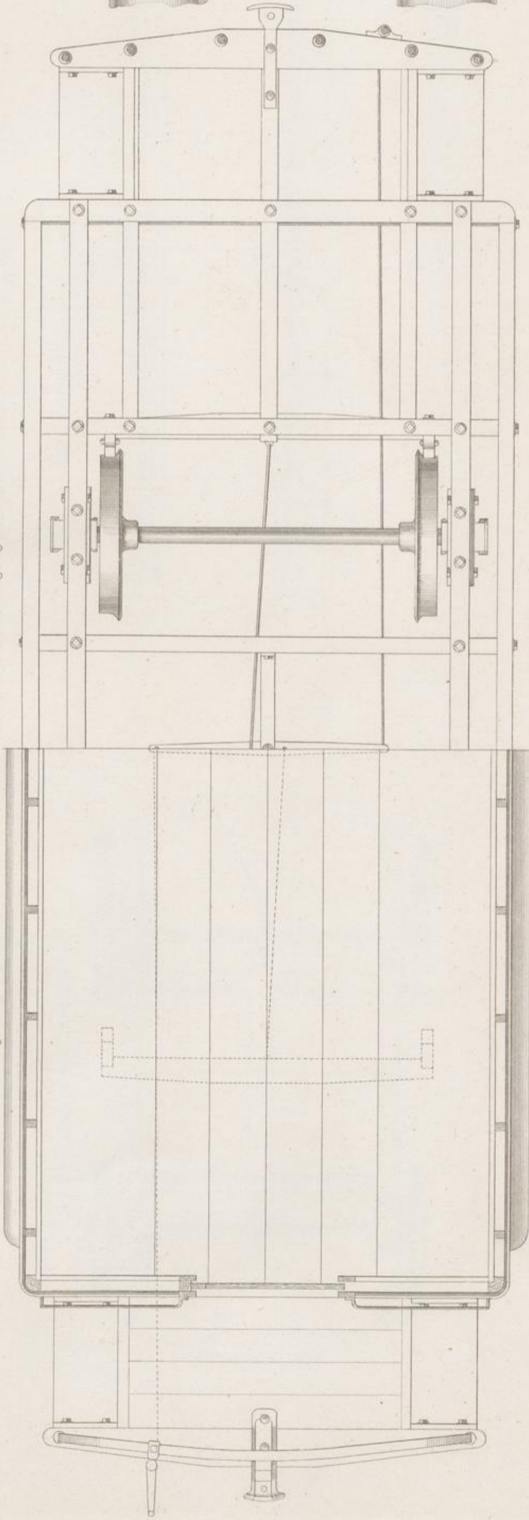
Fig. 3 Horizontalschnitt über den Sitzen u. Oberansicht des Wagenstellens
