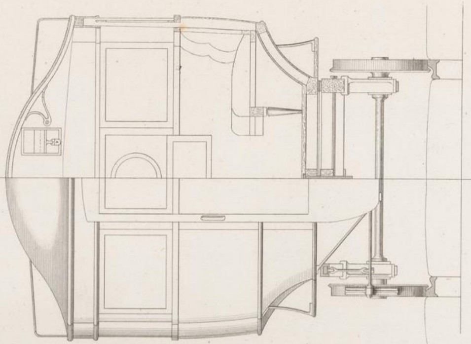
Fig. 3 Hinteransicht Querschnitt
