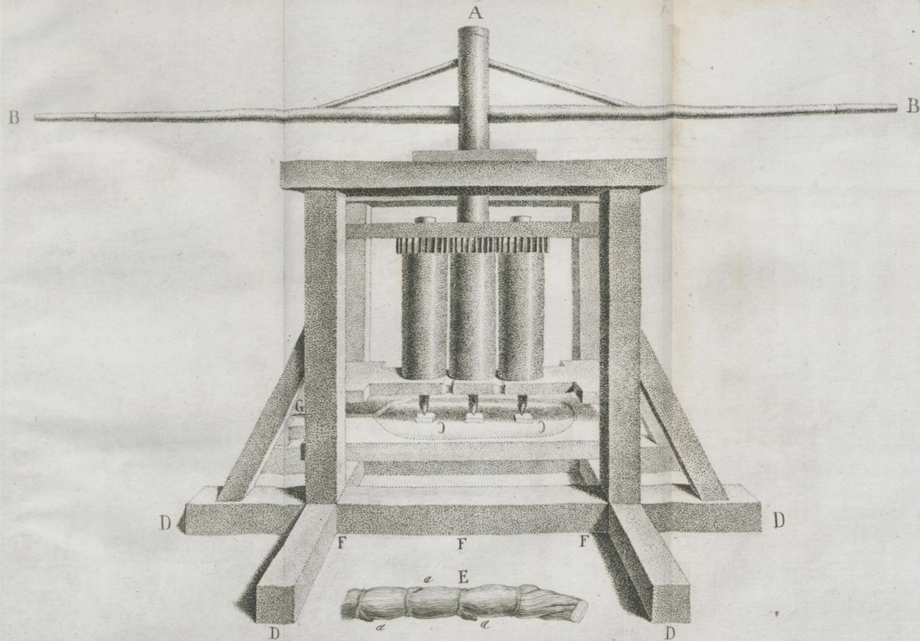
Motino per comprimere le Canne Zuccherine
