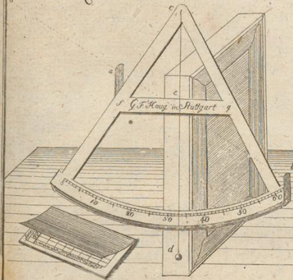
Ein holzener Sextant
