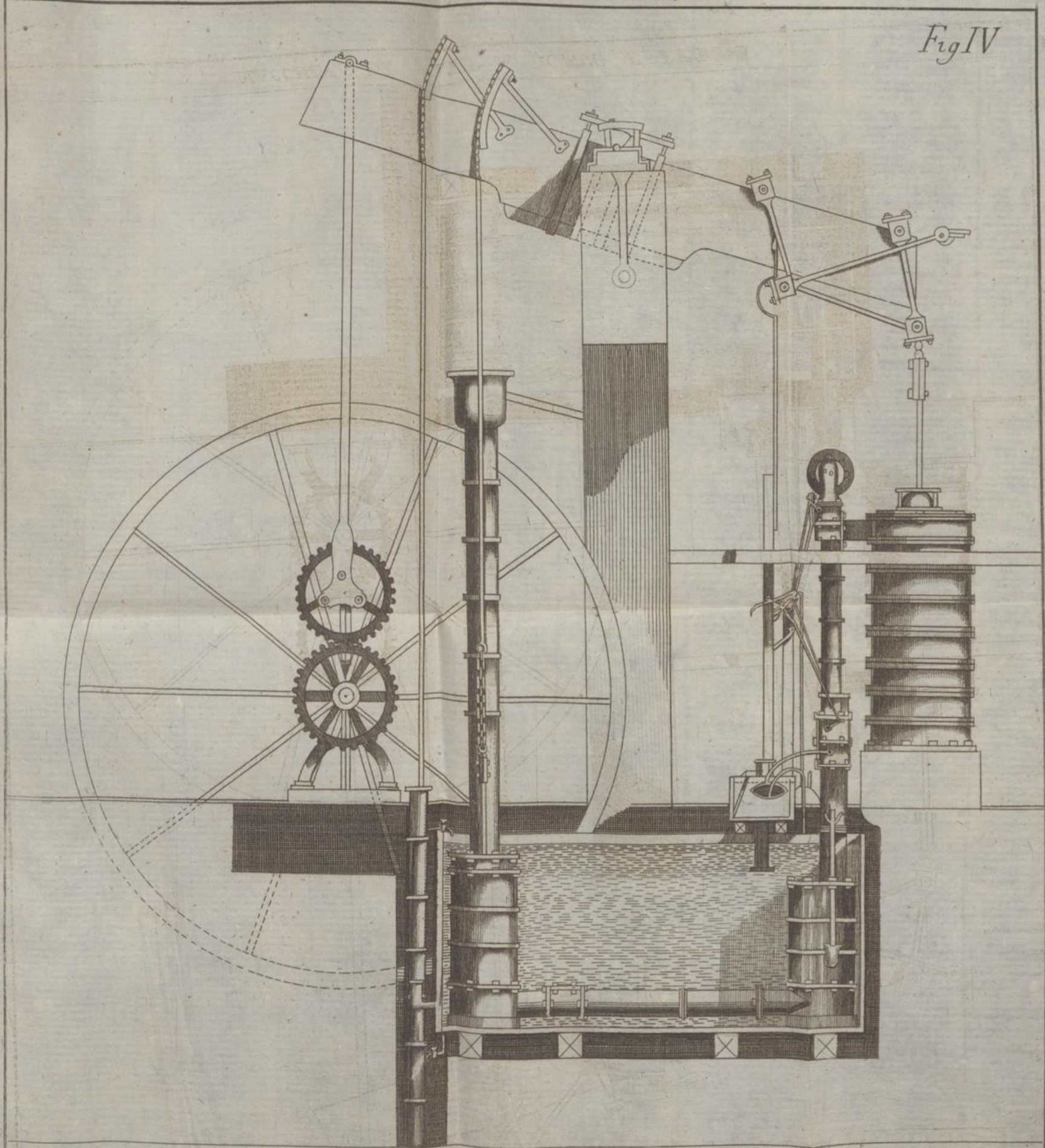
MACCHINA DI WATT A DOPPIO EFFETTO
