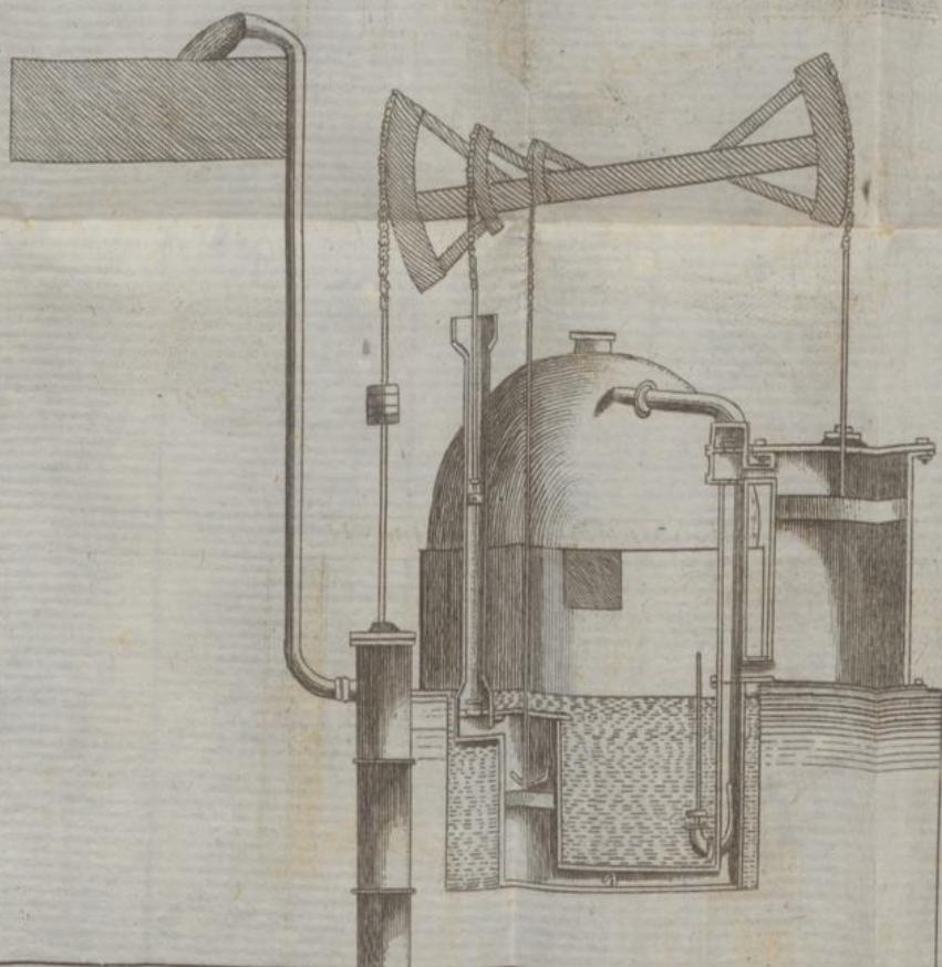
MACCHINA DI WATT
