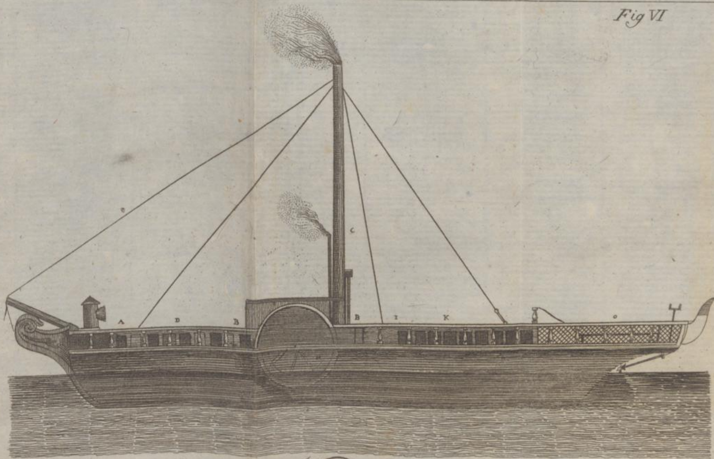
L' ETNA Nave a Vapore Prospetto
