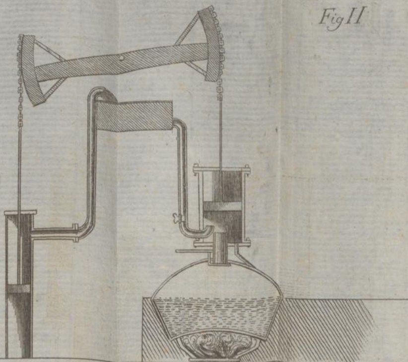
MACCHINA DI NEWCOMEN
