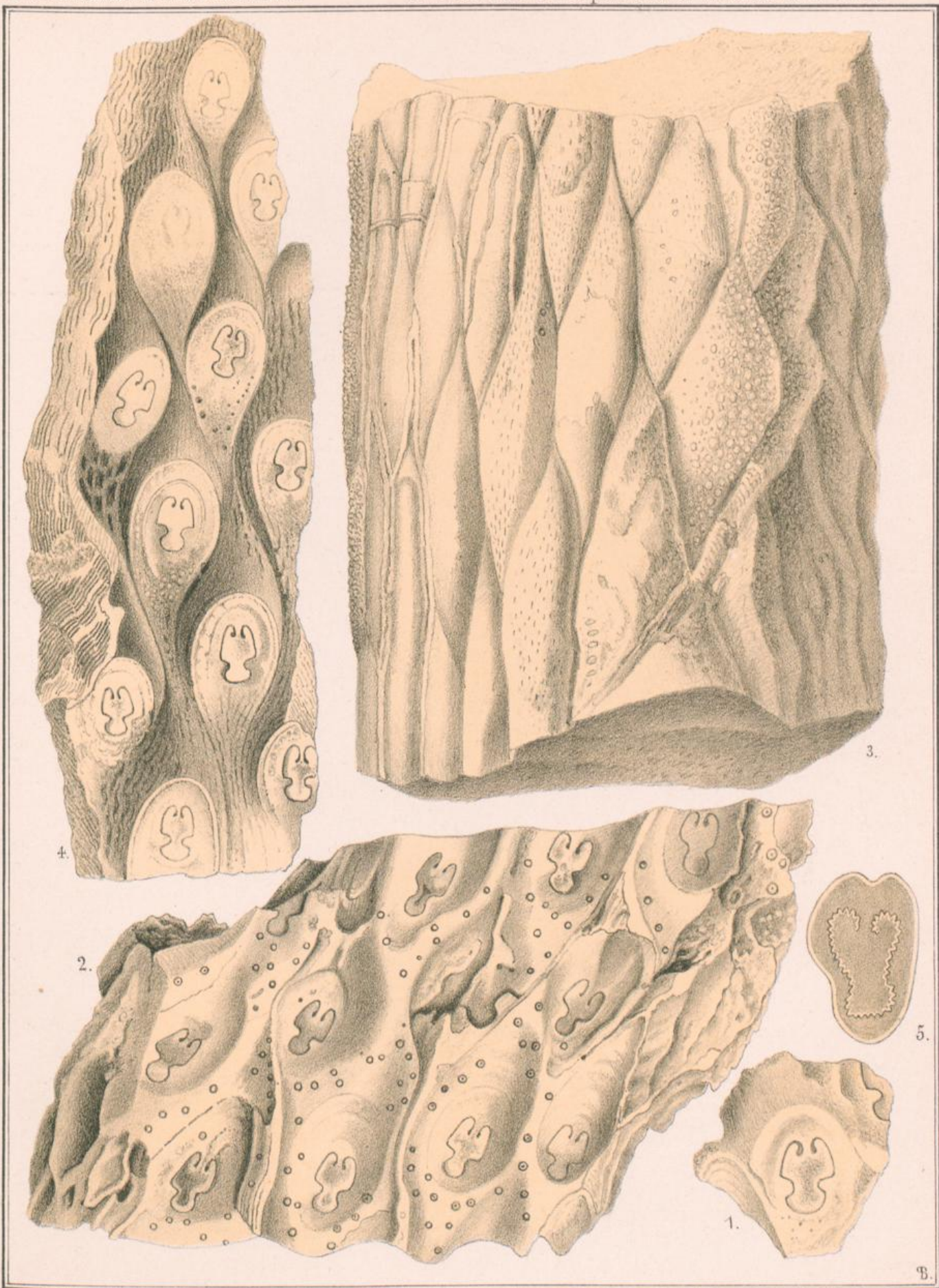
Protopteris punctata.
