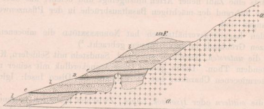
a. Horizontale Lager von Basalt und Basaltstuf. b. Sand und weicher Sandstein. c. Kleine, unregelmässige Kohlenlager. D. Sandiger Schiefer mit Pflanzenresten.
