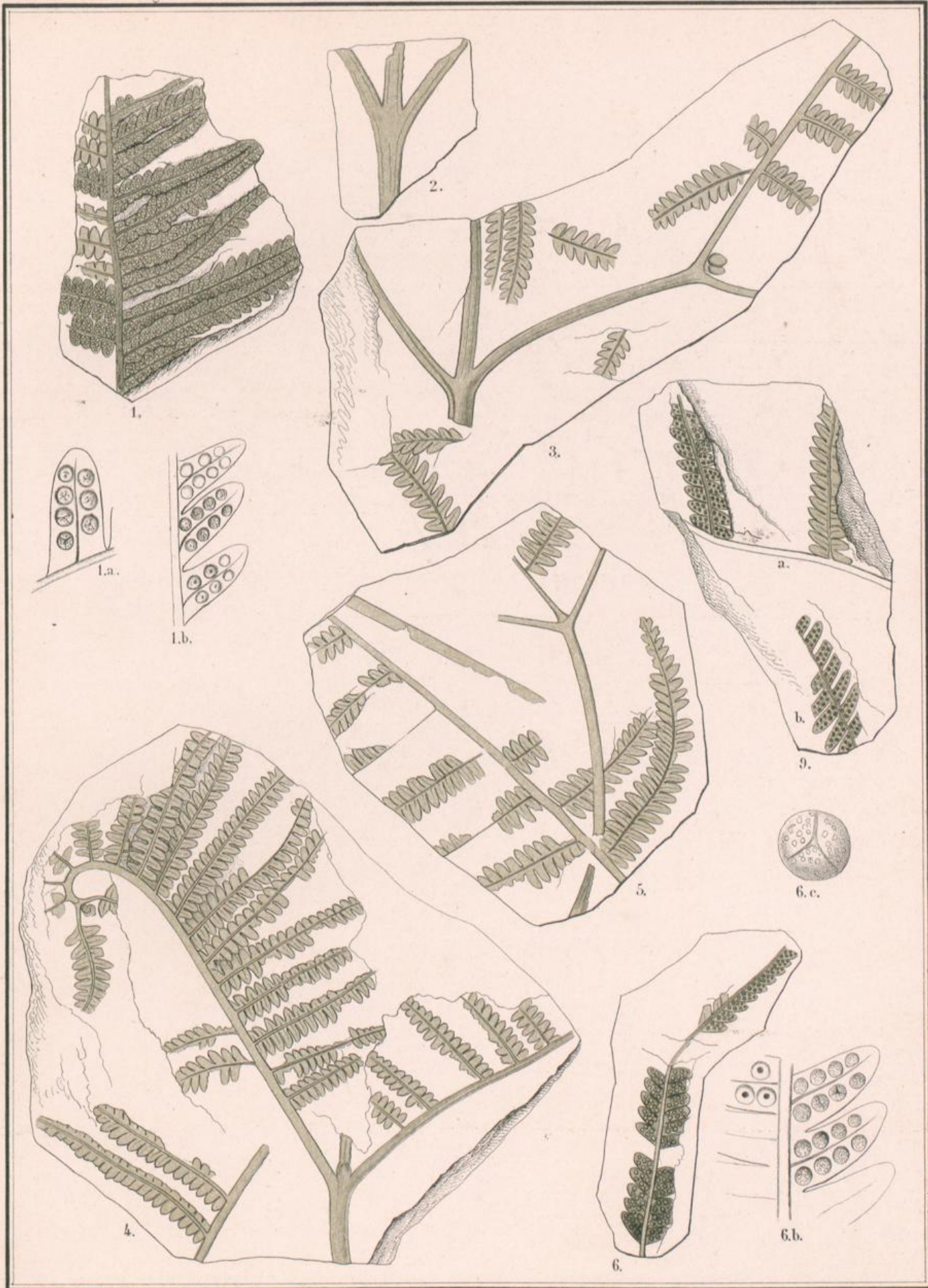
Gleichenia Zippii.
