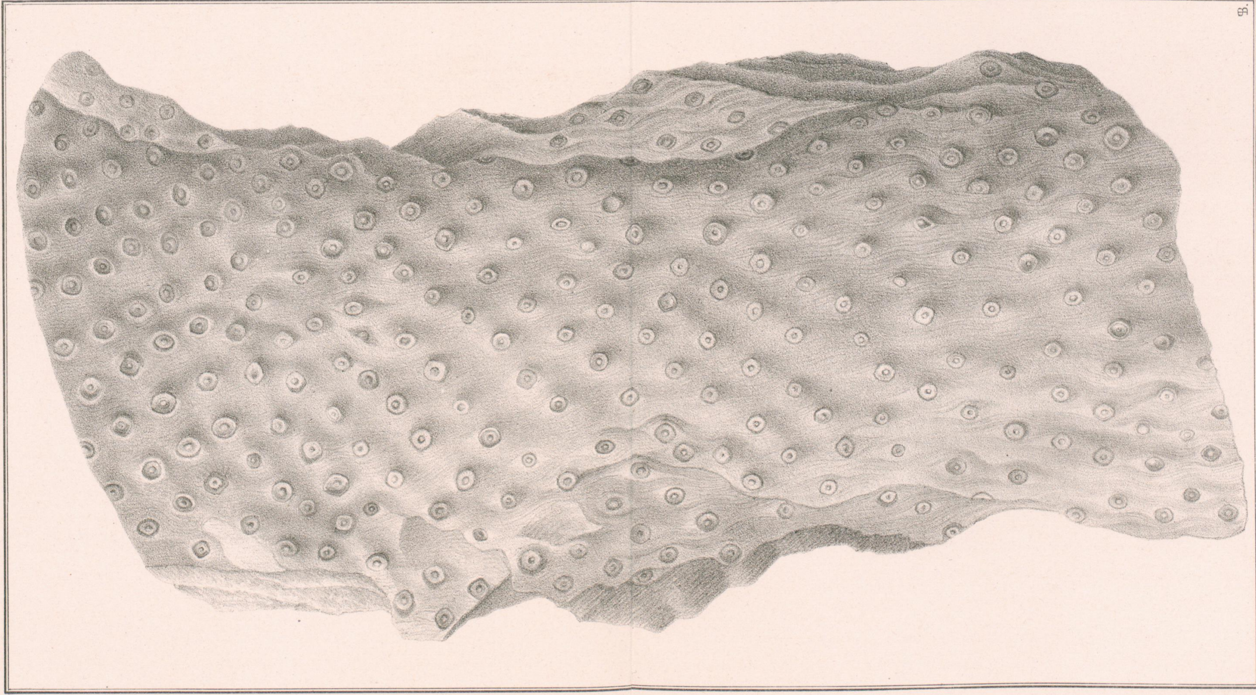
Stigmaria.
