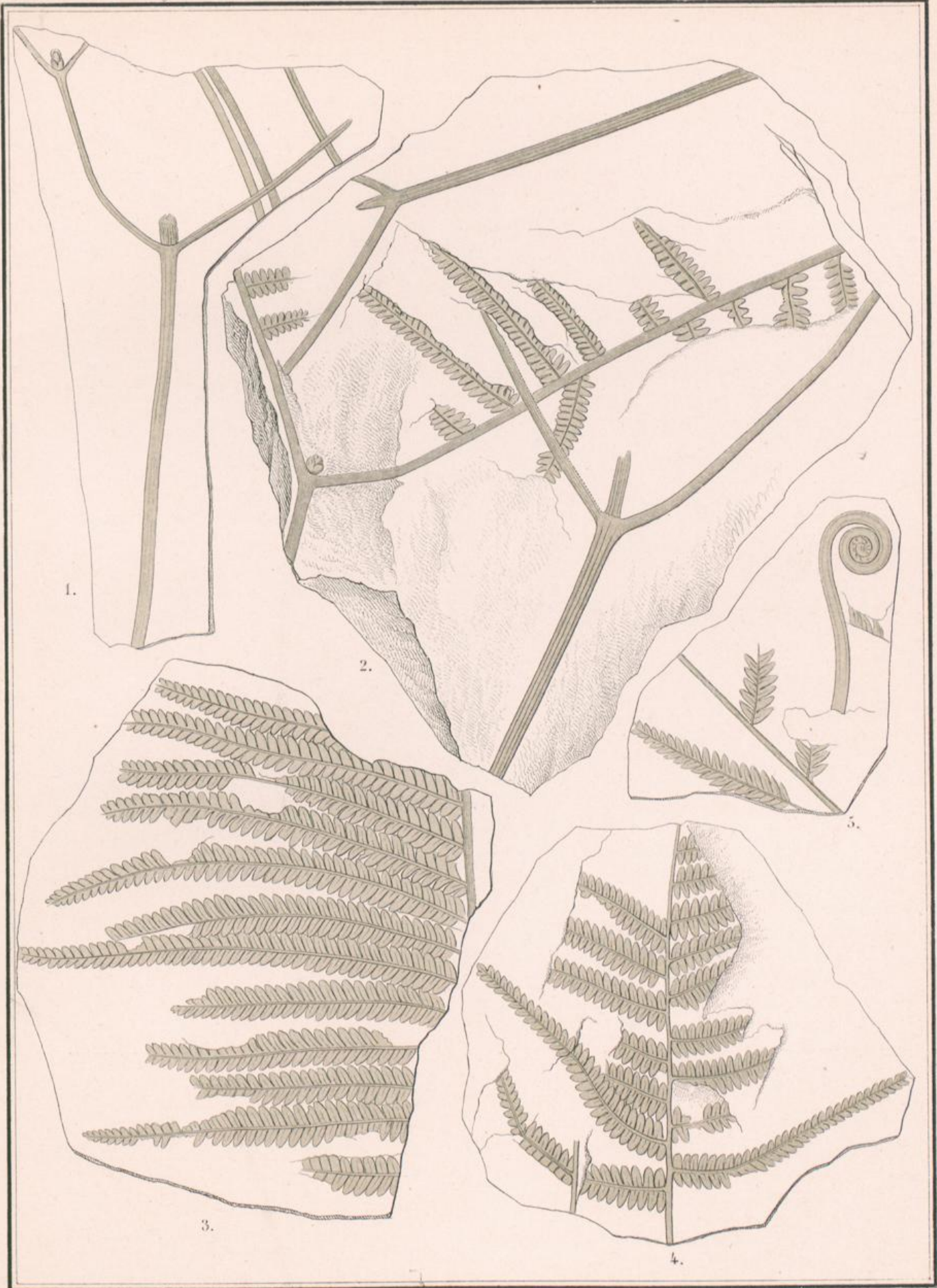
Gleichenia Zippelii .
