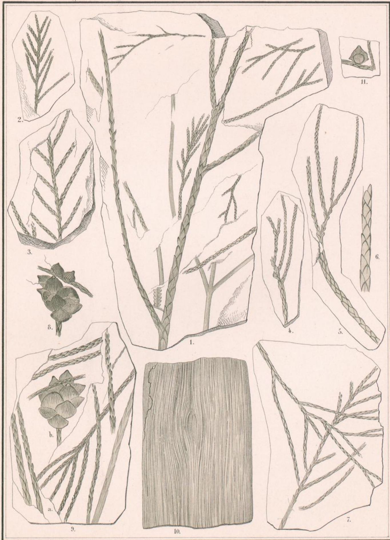
Cyprissidium gracile.
