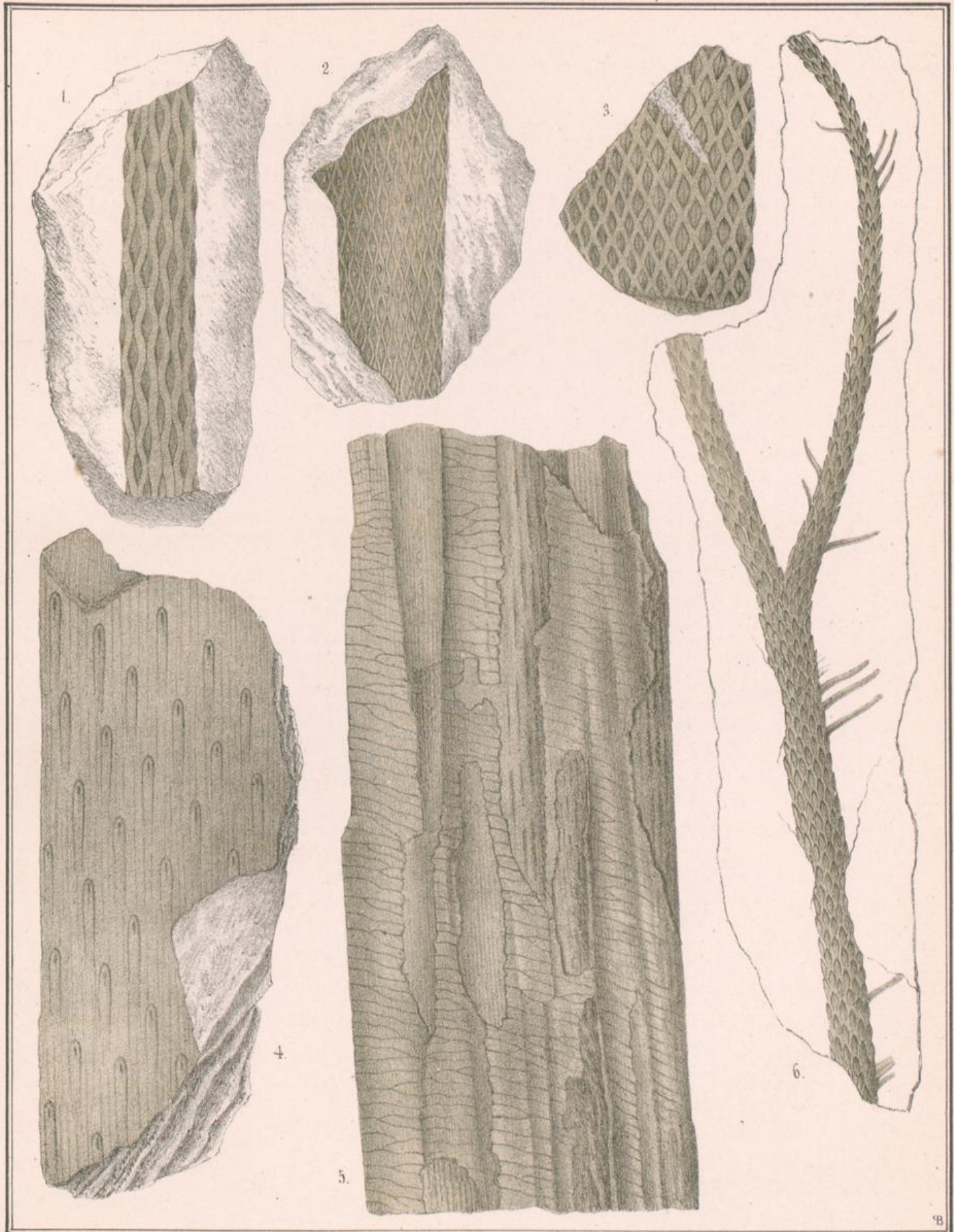
Lepidodendron Veltheimianum.
