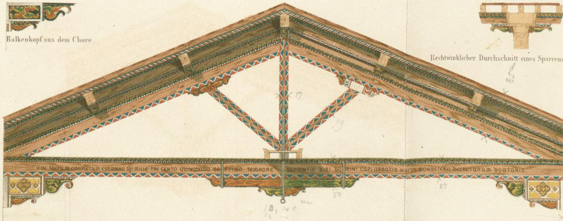
Maasstab in \frac{1}{40} der wahren Grosse.
