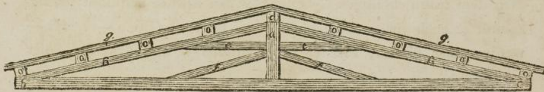
Fig. 1. Zimmerwerk.
