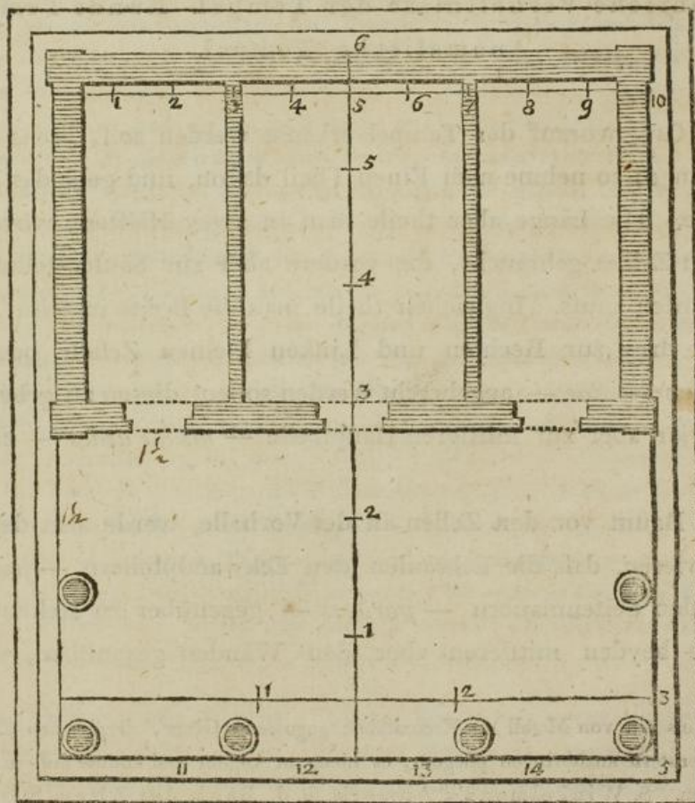
Fig. 2. Toskanischer Tempel.
